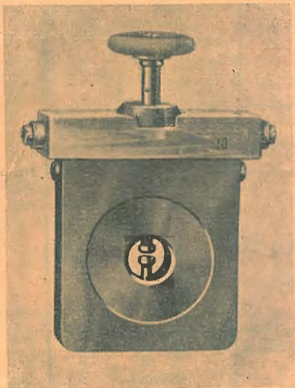
Fig. 1 - Cellula Karolus per ricezione.
